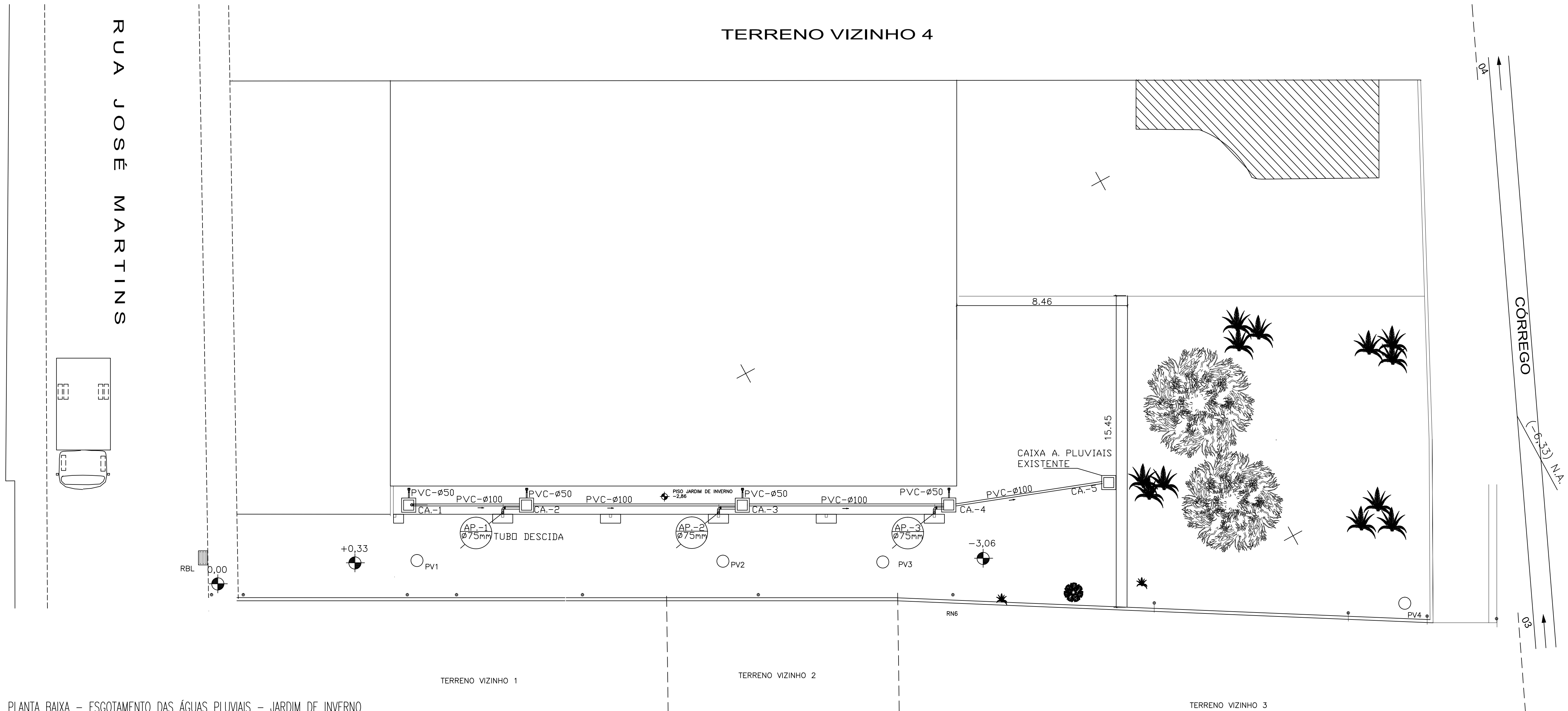
PLANTA BAIXA – ESGOTAMENTO DAS ÁGUAS PLUVIAIS – JARDIM DE INVERNO Escala: 1: 50
