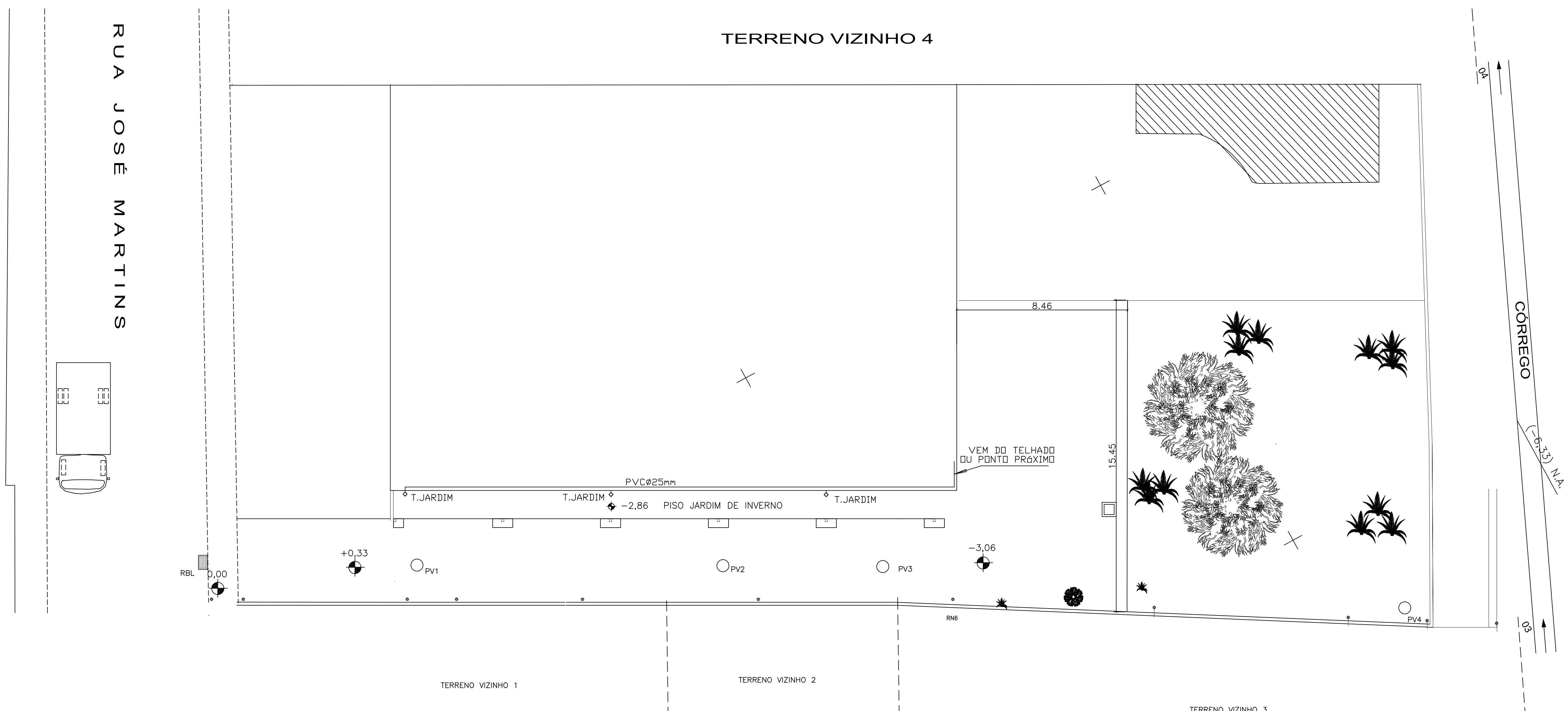
PLANTA BAIXA – ALIMENTAÇÃO DE ÁGUA – JARDIM DE INVERNO Escala: 1: 50
